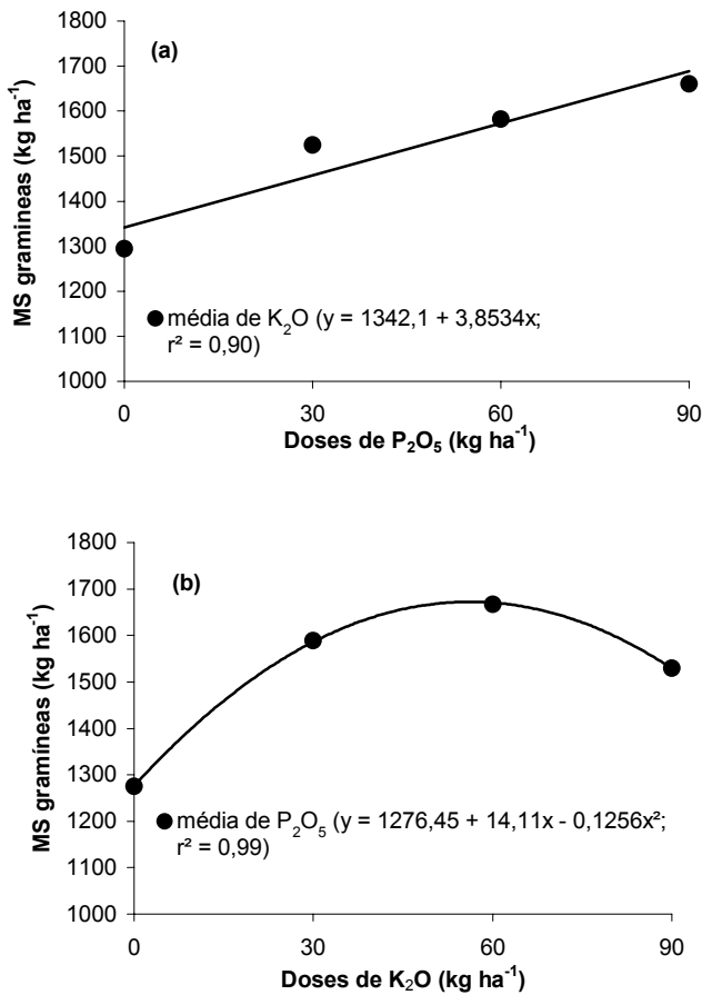
Figura 4 - Rendimento de matéria seca de gramíneas na média das doses de fósforo (a) e na média das doses de potássio (b). Pelotas/RS, 2001/2002.
