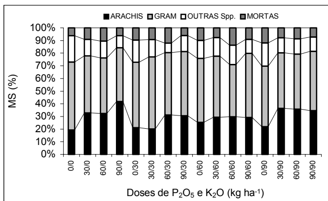
Figura 5 - Porcentual das frações amendoim-forrageiro, gramíneas, outras espécies e material morto no rendimento de matéria seca. Pelotas/RS, 2001/2002
