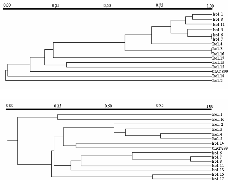
Figura 3. Agrupamento das sequências REP (a) e ERIC (b) de isolados de rhizobium , com determinação de similaridade pelo coeficiente Simple Matching (SM) e método de agrupamento UPGMA.
